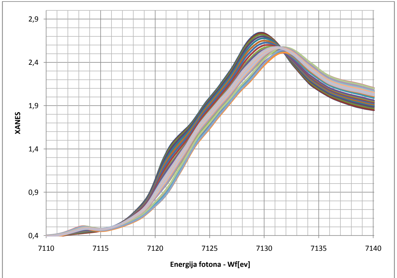
Graf spektrov XANES
