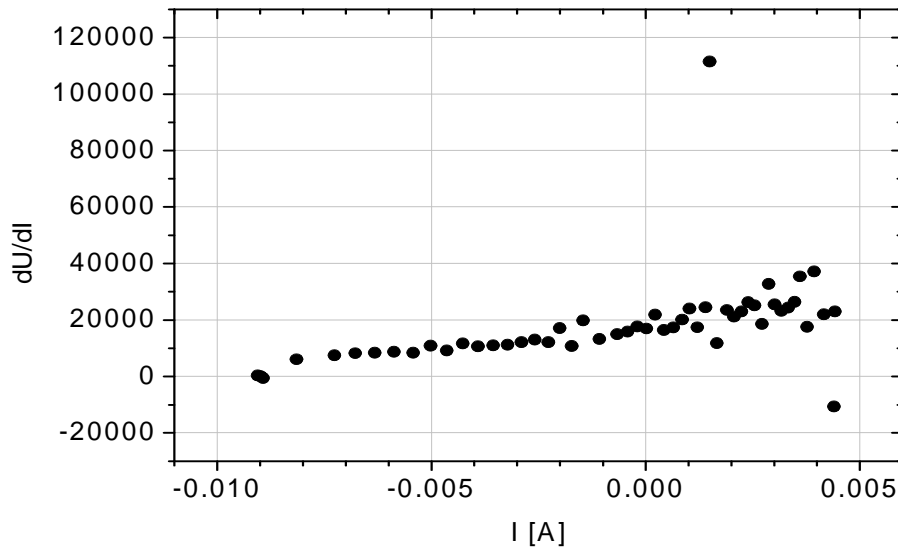
Diferencialna upornost dU/dI za tokovno odvisnost v datoteki "Korozija.dat"
