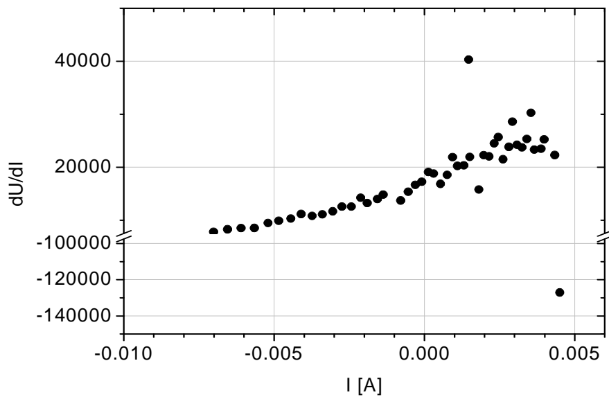
Diferencialna upornost dU/dI za tokovno odvisnost v datoteki "Korozija.dat"
