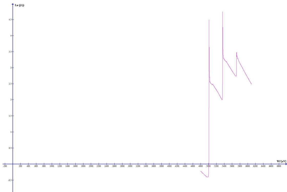
Graf 3: absorpcija rentgenskih žarkov v cezijevi pari
