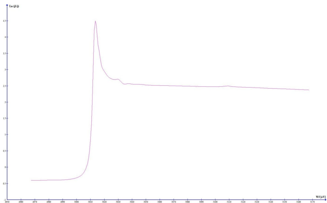
Graf 4: absorpcija rentgenskih žarkov v cezijevi pari, v območju roba L3
