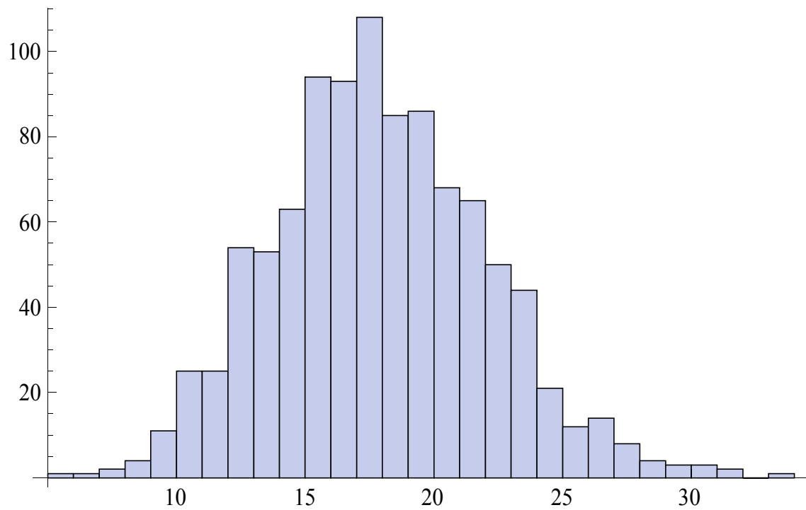
Histogram 1: Število radioaktivnih razpadov šibkega izotopa
