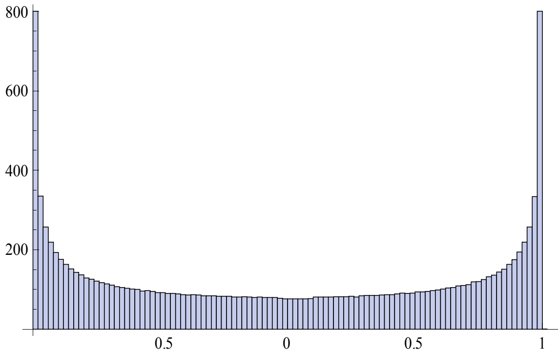
Histogram 4: sinusna funkcija
