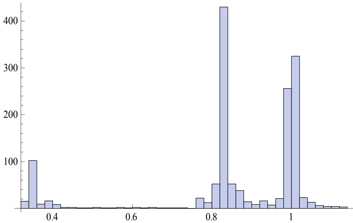
Histogram 3: absorpcijski spekter
