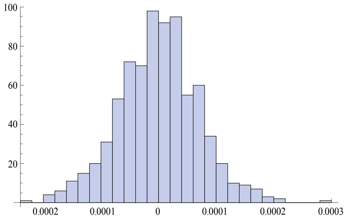
Histogram 2: meritev absorpcije rentgenskih žarkov
