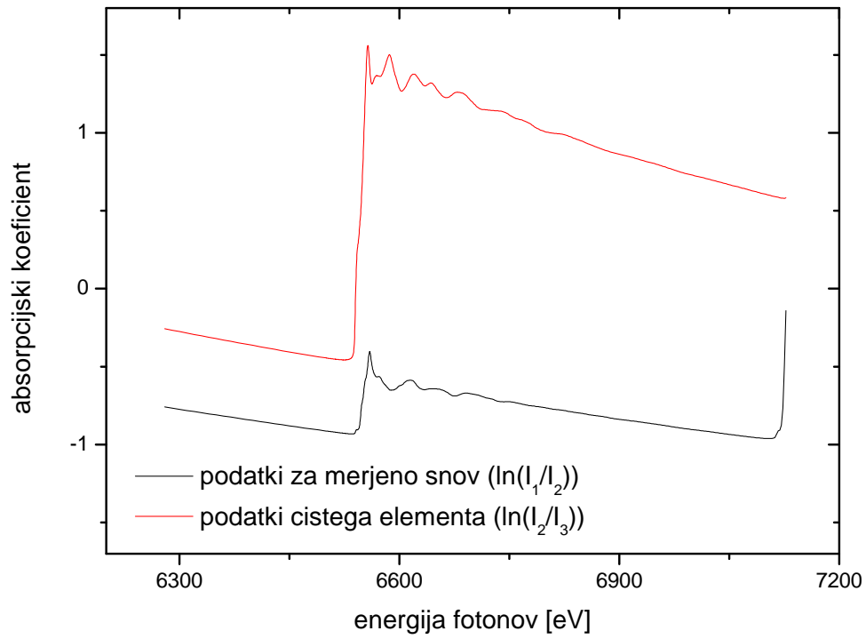
graf meritev absorpcijskega koeficienta neznane snovi in čistega elementa
