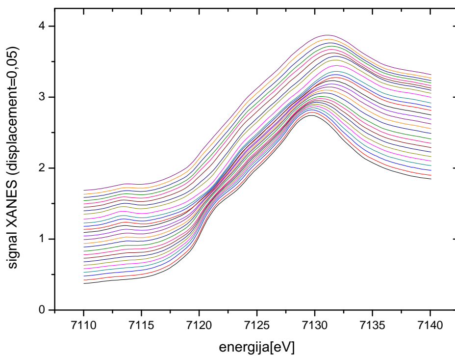
graf spektrov K železa v li-ion bateriji med polnjenjem in praznjenjem
