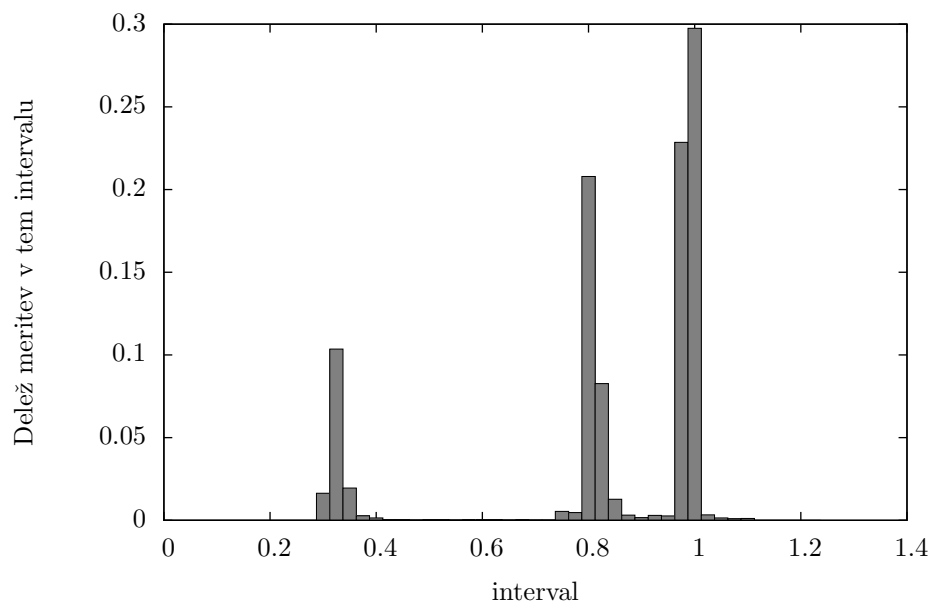
Absorbcijski spekter
