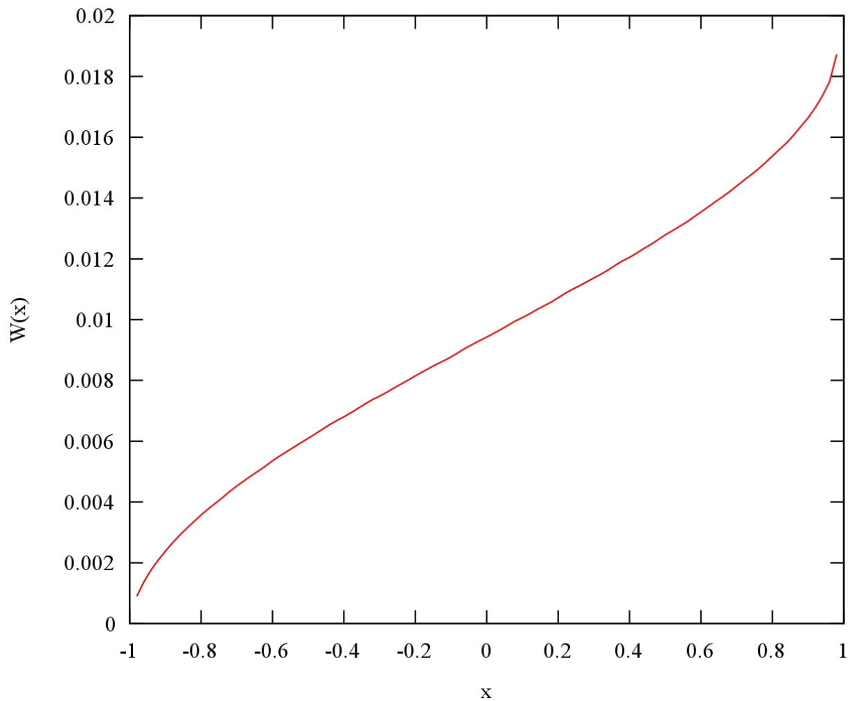
Graf: Integralska verjetnost porazdelitve sinusne funkcije
