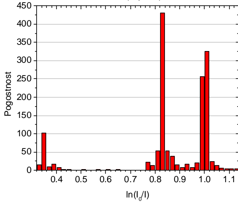
GRAF 3: Absorpcijski spekter EXAFS
