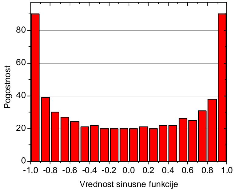
GRAF 4: Histogram sinusne funkcije
