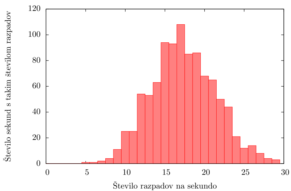
Radioaktivni razpadi šibkega izotopa
