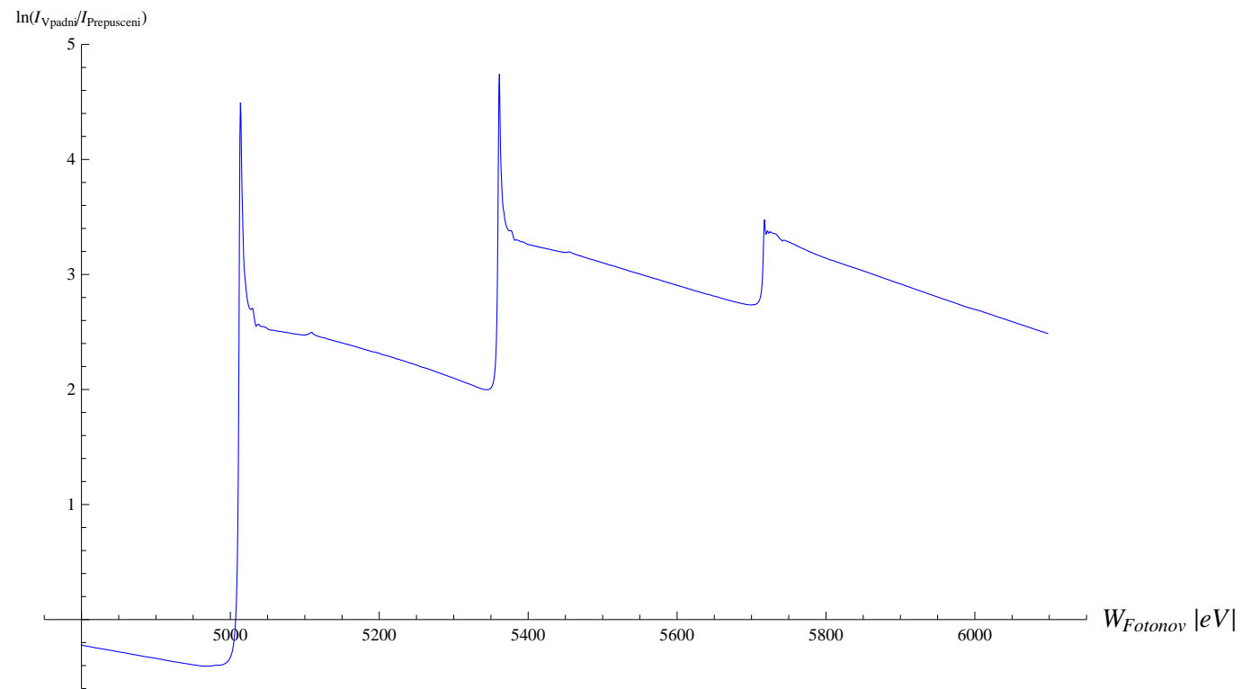
graf meritve absorbcije rentgenskih zarkov
