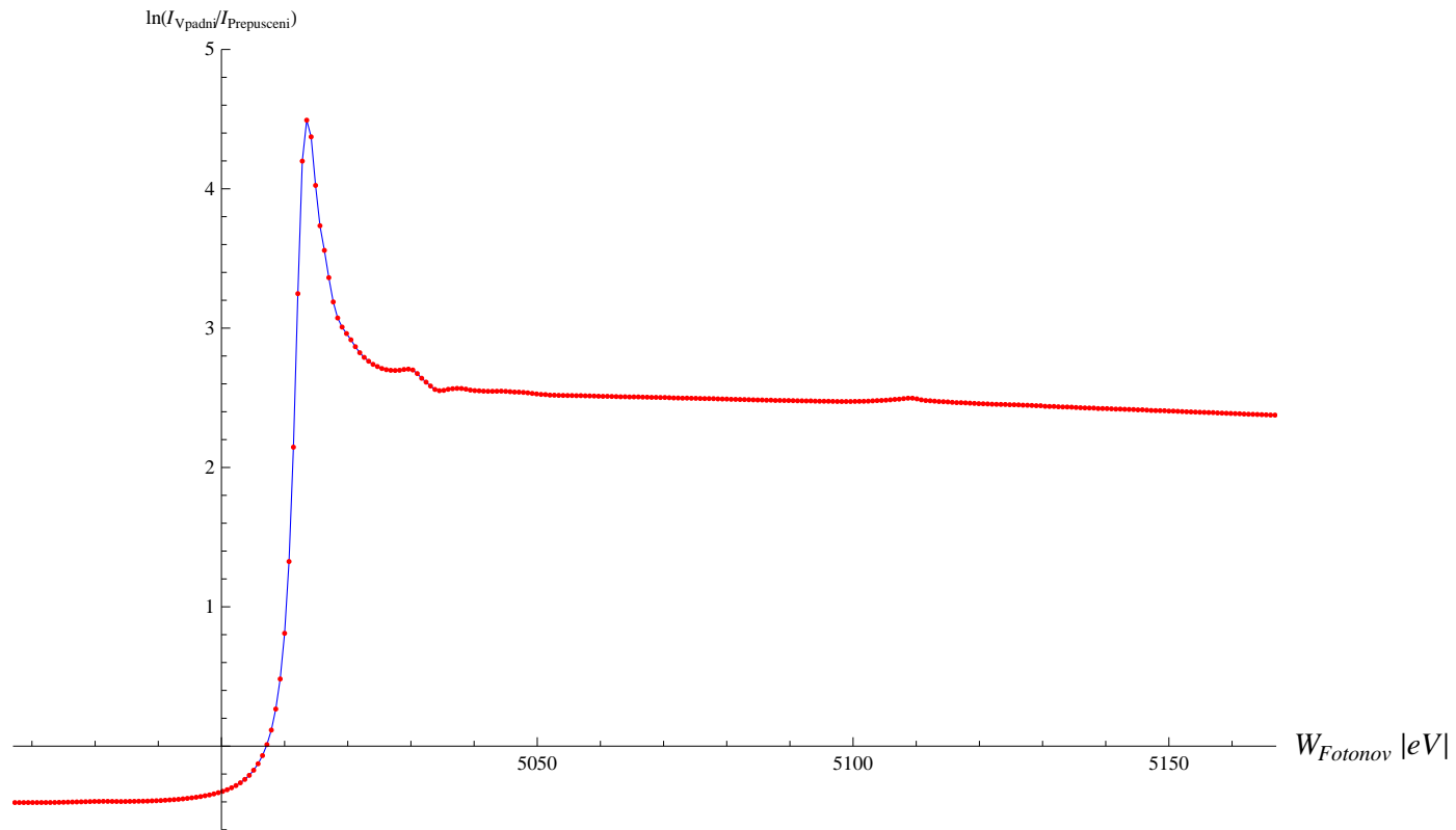
graf meritve absorbcije rentgenskih zarkov – povecano
