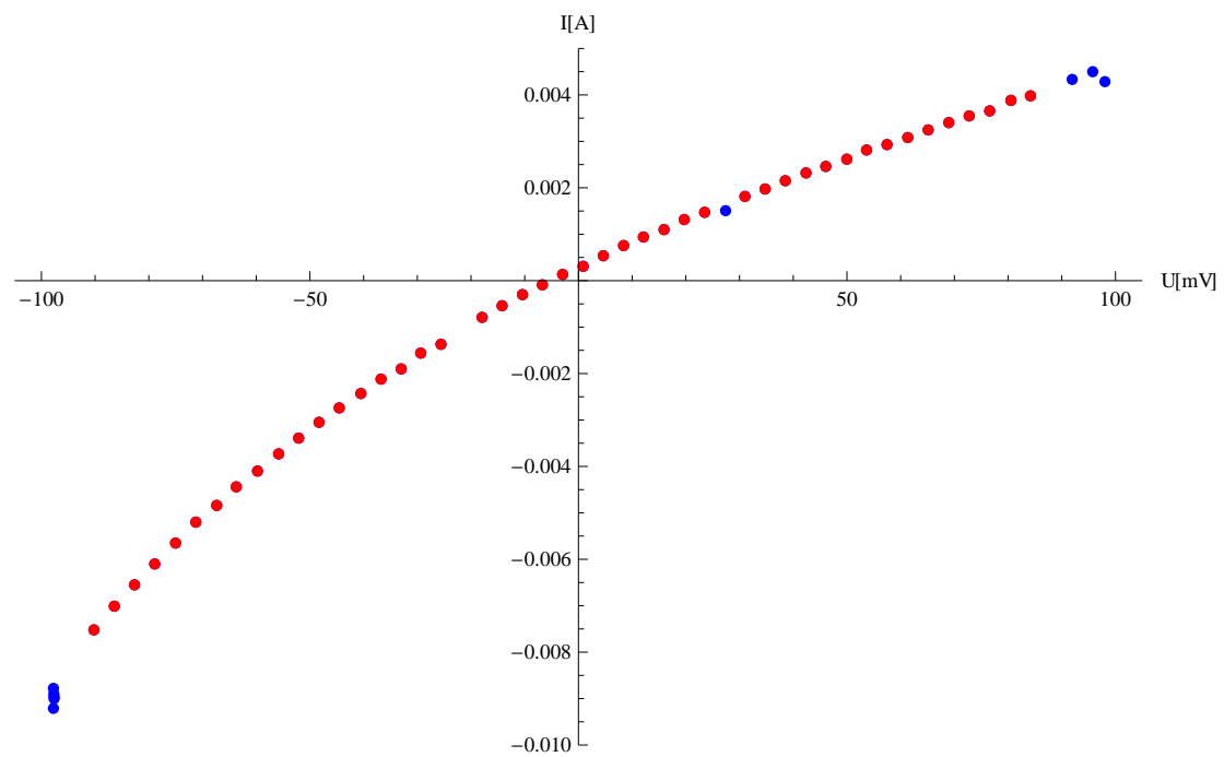
karakteristike I–U za kovinsko elektrodo
