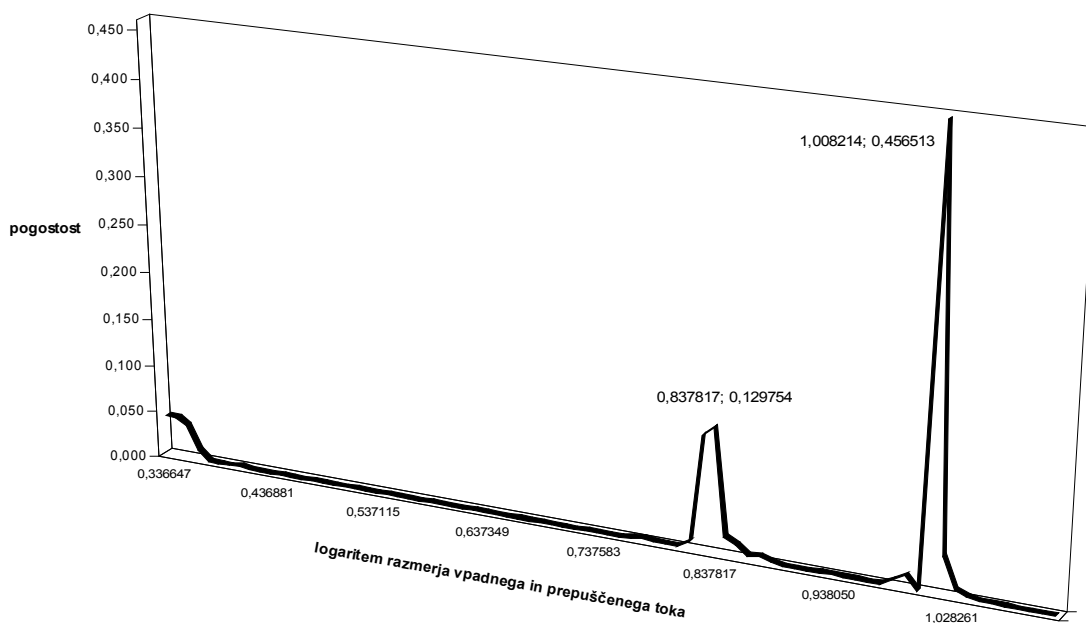
absorpcijski spekter EXAFS (Extended X-ray Absorption Fine Structure = drobna struktura rentgenskih absorpcijskih robov) mešanega železovo-kobaltovega oksida
